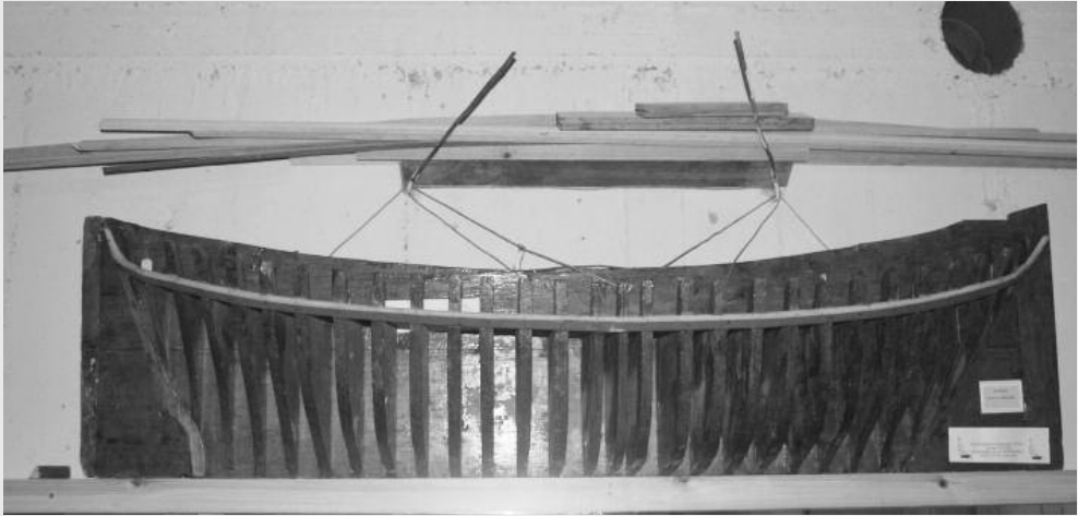
Το μισομόδελο του περάματος «Φίλιππος» κατασκευασμένο το 1948 από τον Εμμανουήλ Γ. Γιαμουγιάννη με ολικό μήκος 18,15 μ.
